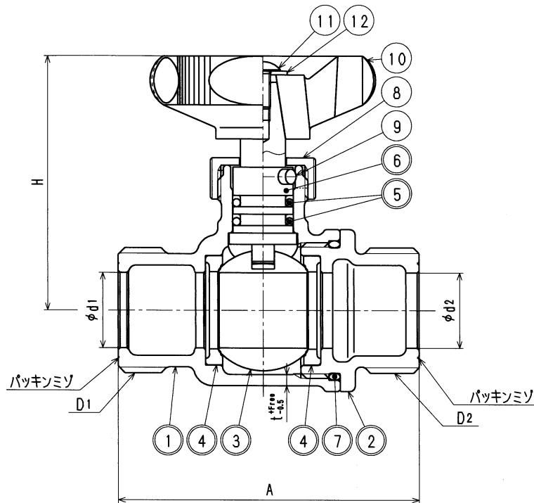
寸法表 (mm)
